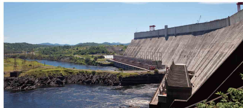
委内瑞拉Guri水电站机组改造工程，装机容量3×300兆瓦+ 3×400兆瓦
